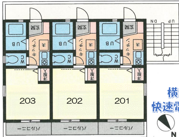
2F 平面図
