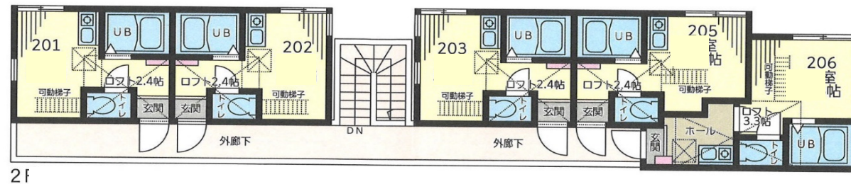
2F 平面図
