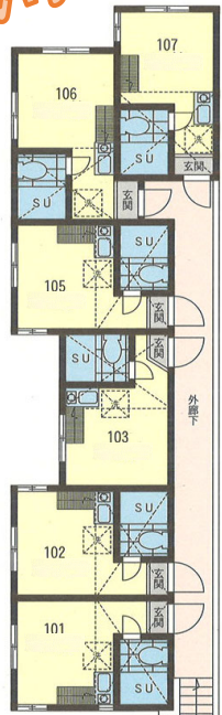
1F 平面図
