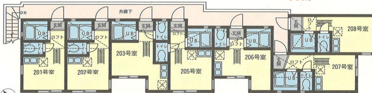
2F 平面図
